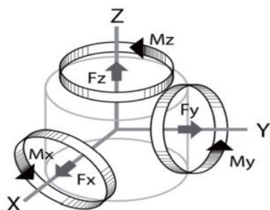
37XX 系列-机器人&amp;通用测试 6 轴力传感器
